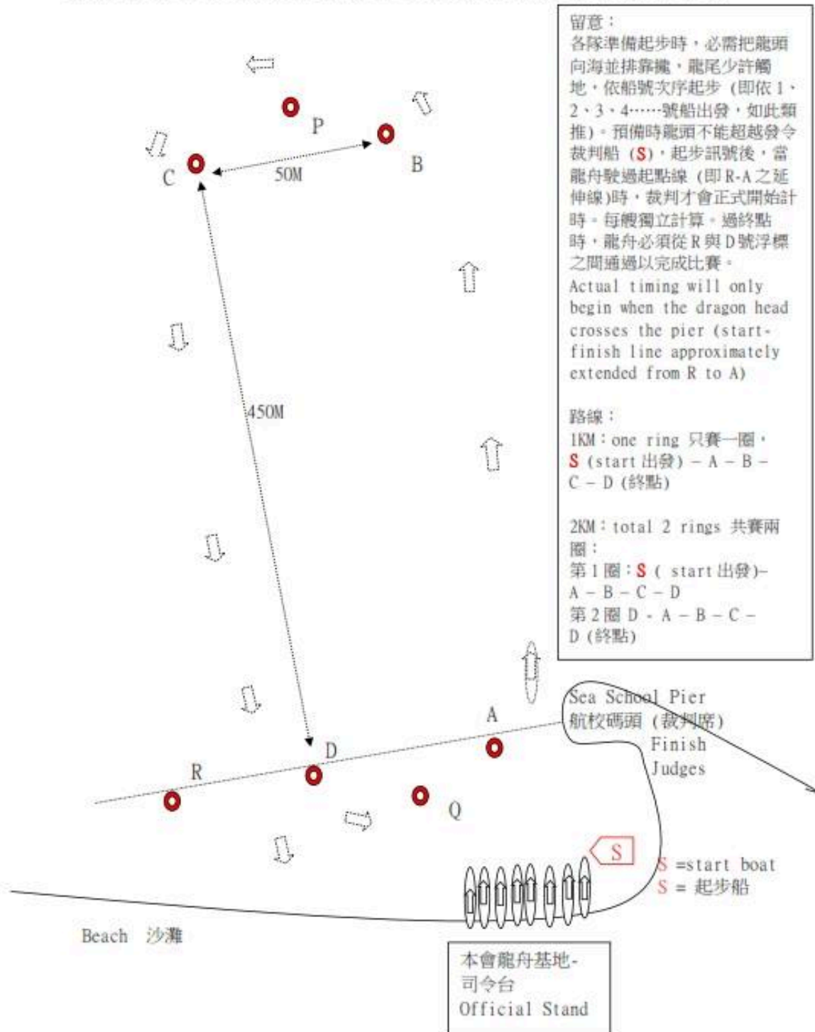
(圖 1) 1000m 及 2000m 環繞追逐賽路線圖 Route for Ring Races
